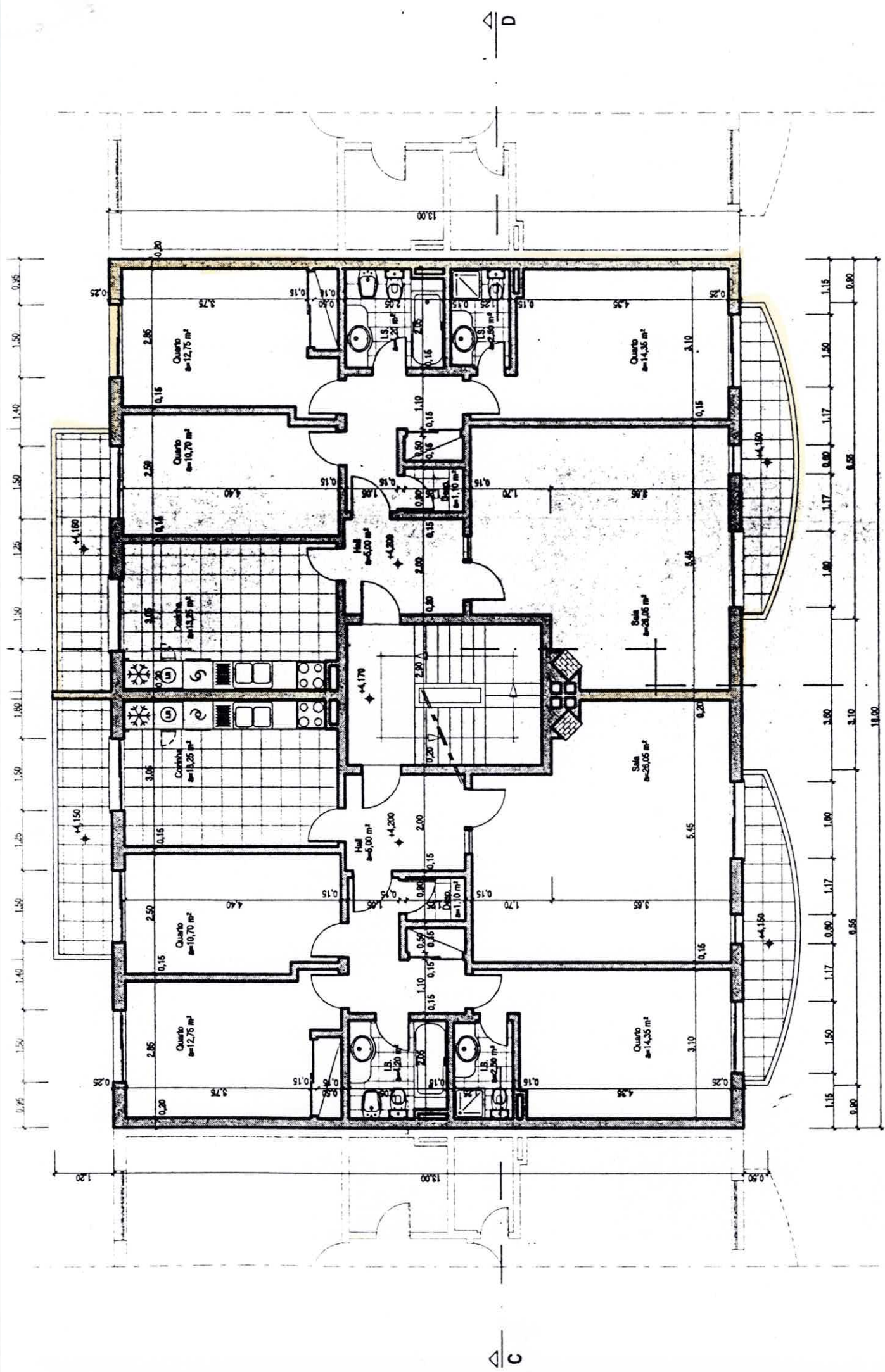
PLANTA DO PISO 1
